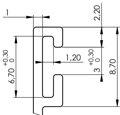
DÉTAIL A ECHELLE 4 : 1
